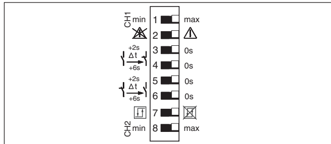
Рис. 3: DIL-переключатель VEGATOR 122
